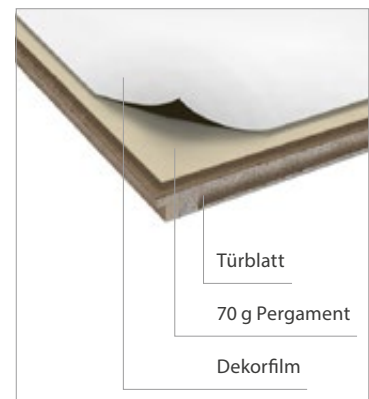
Detail Oberflächenaufbau
